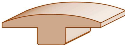
T-Mould 7710 * \frac{5}{8} \times 2
